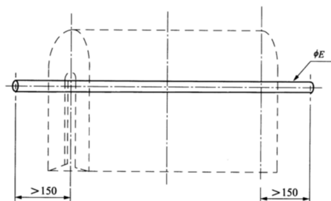
a) 硬质导线遮蔽罩电极
