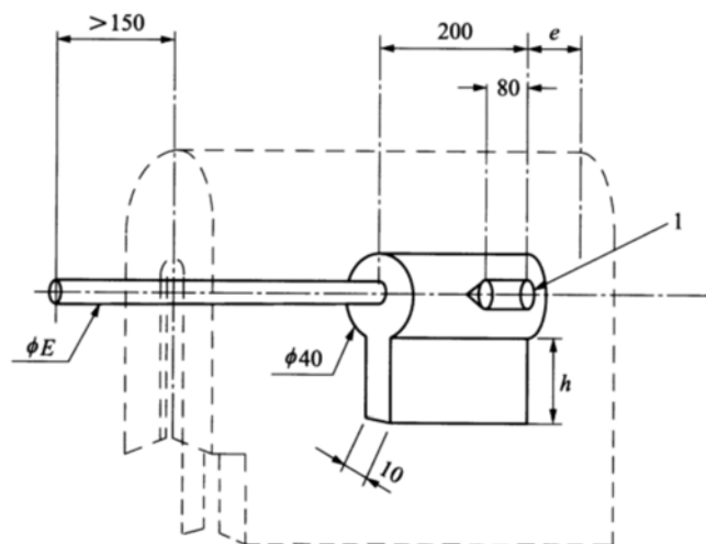
b) 耐张装置遮蔽罩的电极
