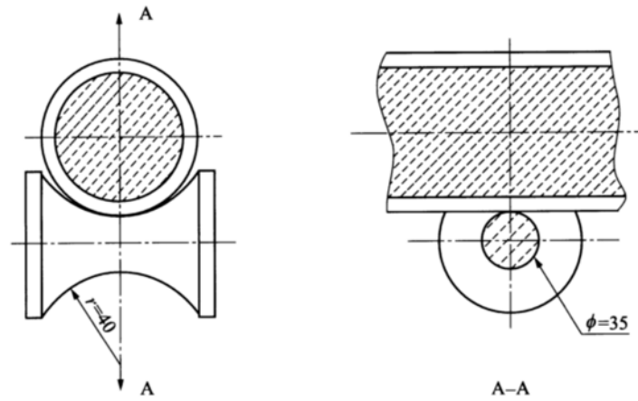
图 C.1 操作杆的弯曲试验布置
