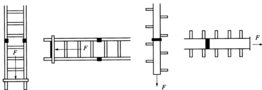
c) 连接装置强度试验布置
