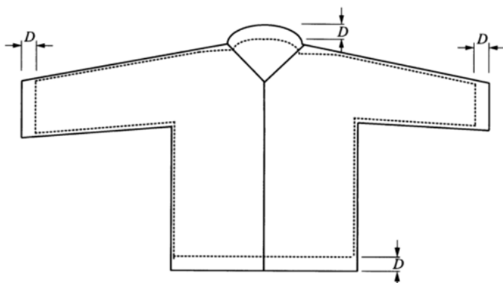
b) 绝缘上衣内电极布置示意图
