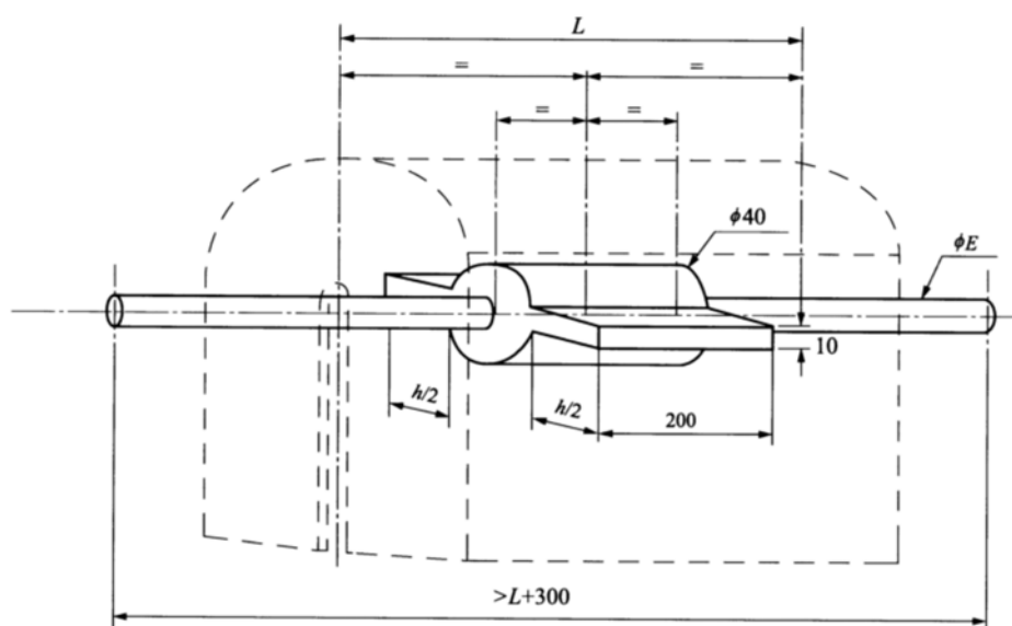
c) 棒形绝缘子遮蔽罩的电极
