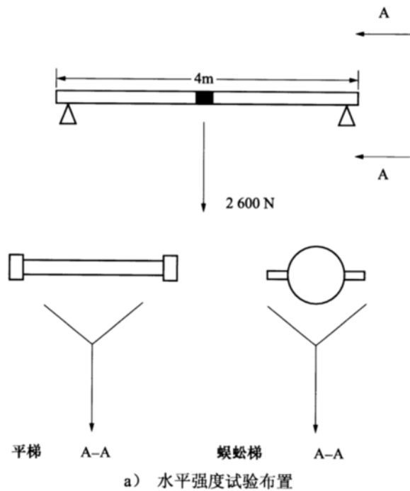
图 C.5 绝缘硬梯的机械强度试验
