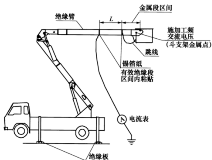
b) 折叠臂式和混合式斗臂车交流耐压试验布置
