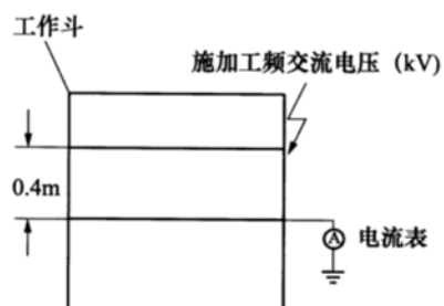
d) 绝缘外斗表面交流耐压和泄漏电流试验
