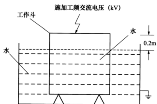
c) 绝缘斗层向耐压试验
