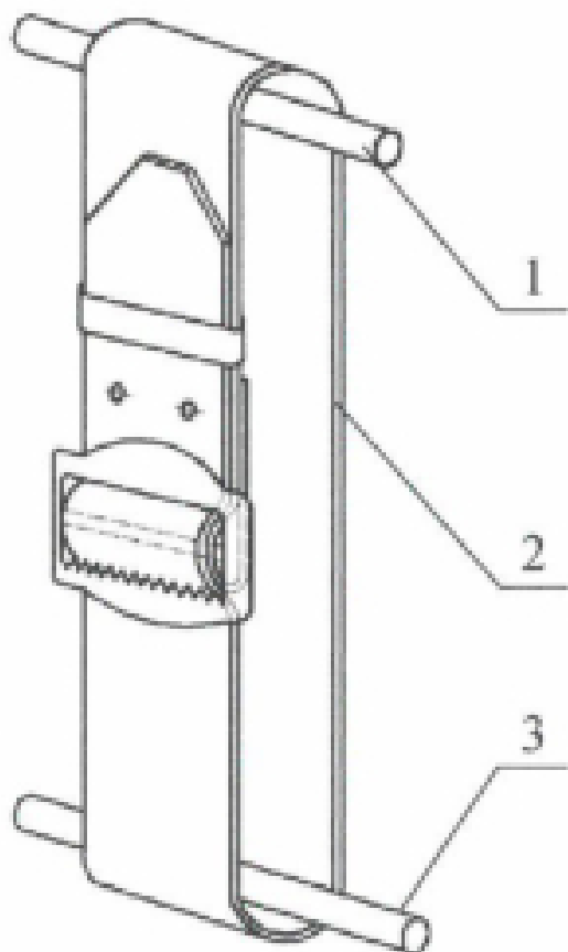
图 C.9 登杆脚扣静负荷试验示意图
