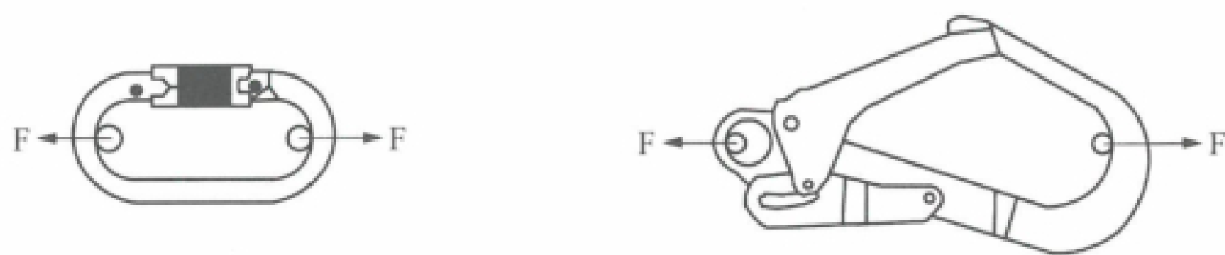
图 C.5 连接器静负荷试验示意图
