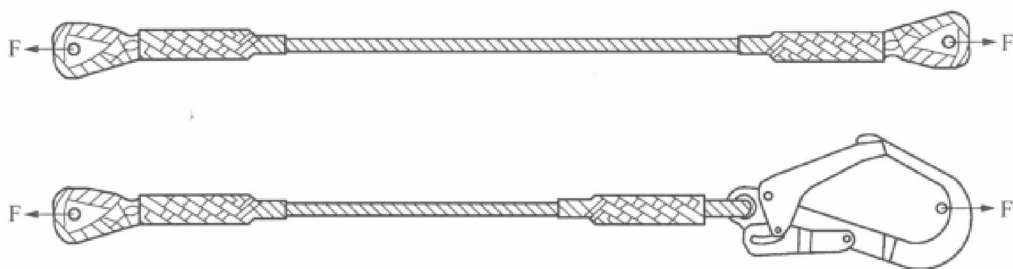
图 C.6 安全绳静负荷试验示意图
