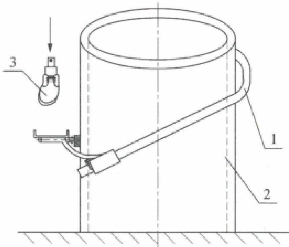
图 C.8 刚性导轨自锁器静负荷试验示意图
