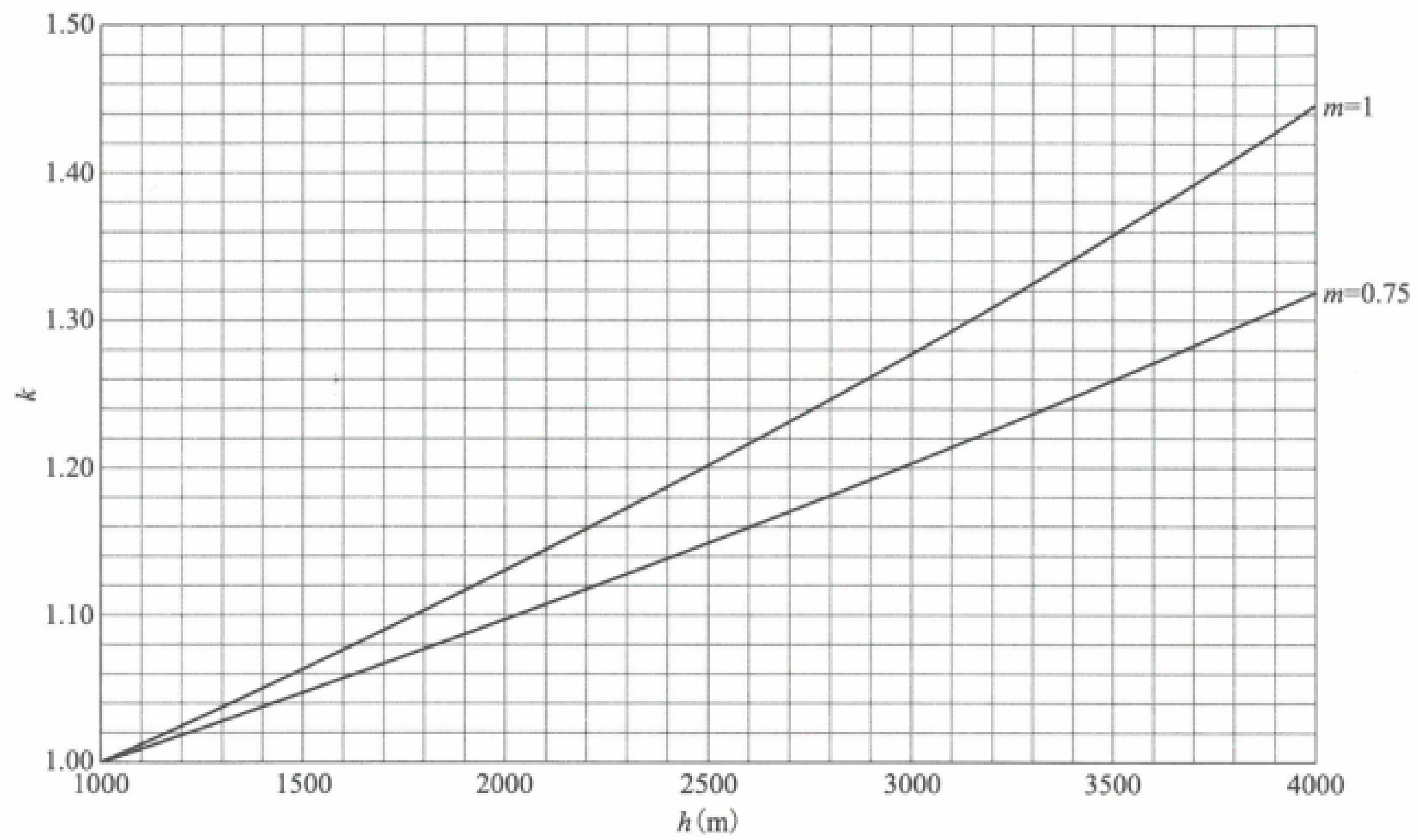
图 A.1 海拔校正因数
