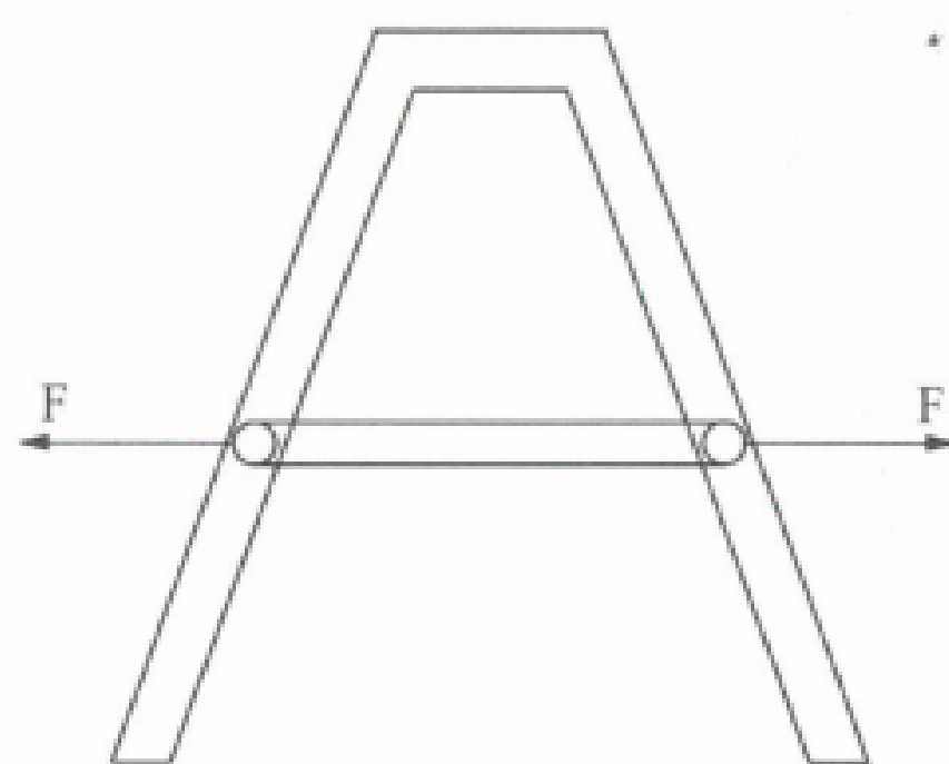
图 C.14 人字梯限张装置强度试验示意图
